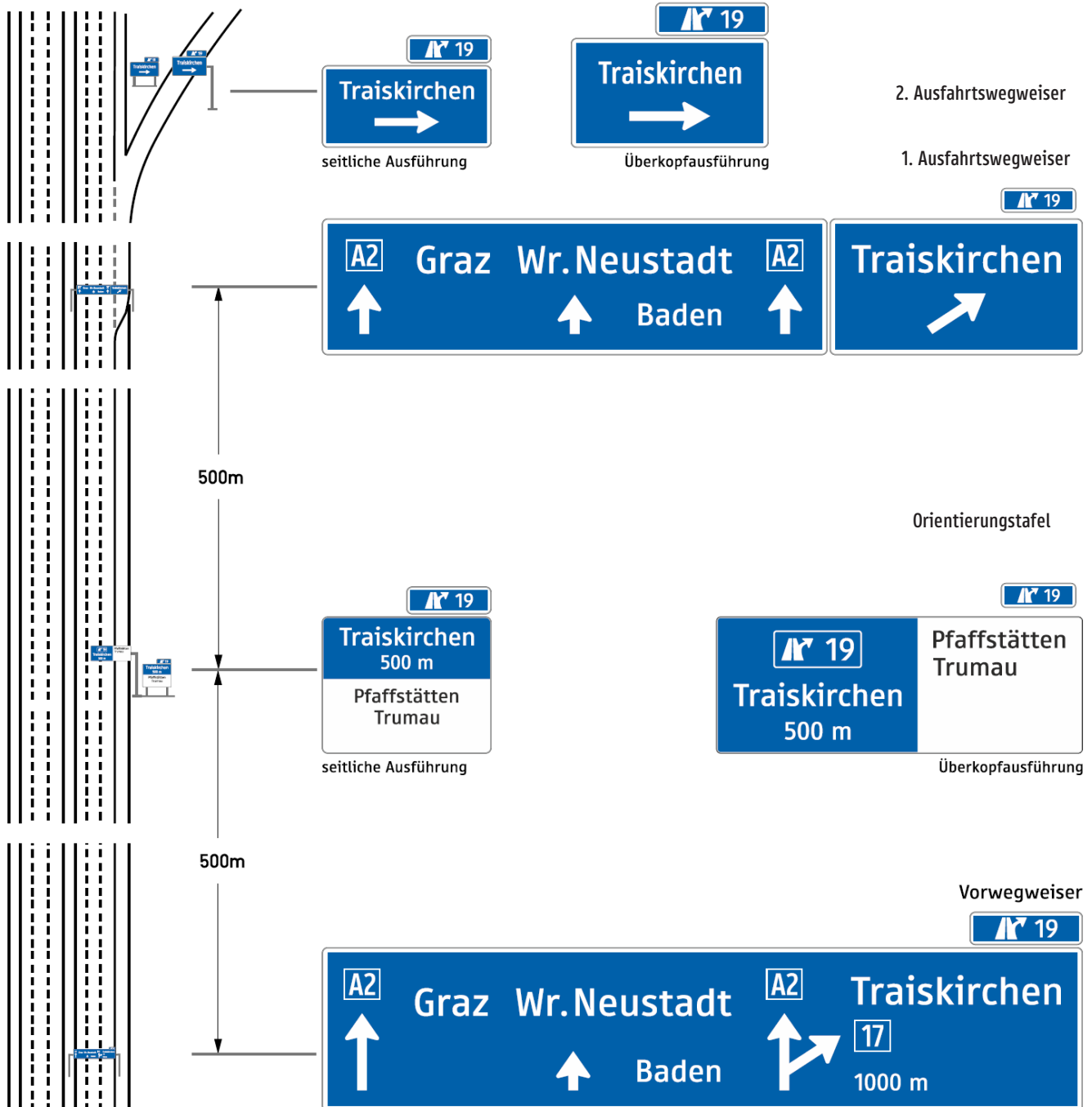
Regelplan Anschlussstelle, RFB mit 3 Fahrstreifen
