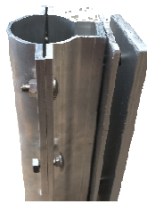
KDE250-Halterung mit 2 Stahlplatten für Befestigung auf Leitschiene
